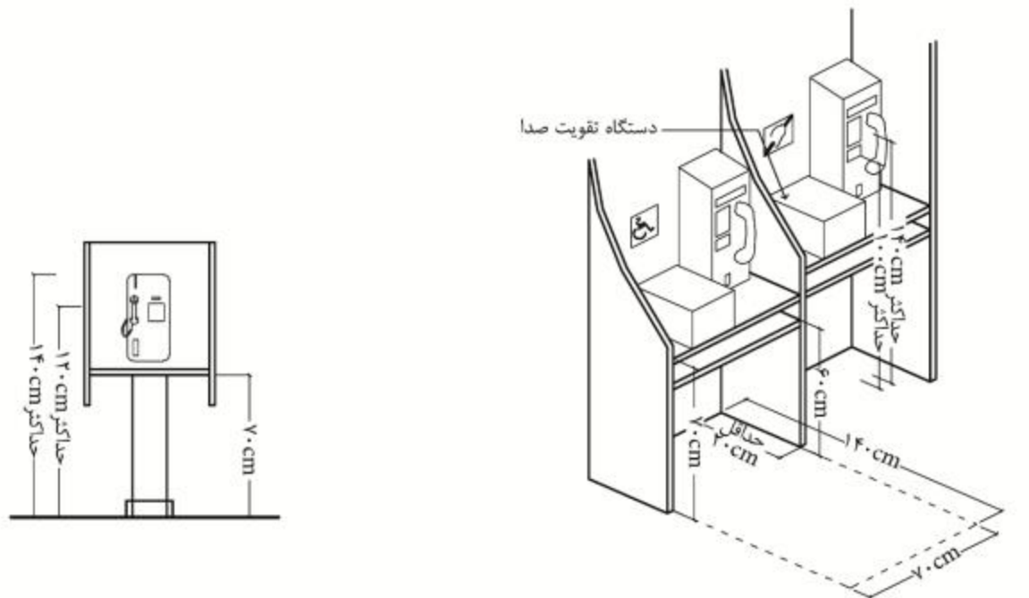
شکل شماره ۴۷: تلفن عمومی دسترس‌پذیر
