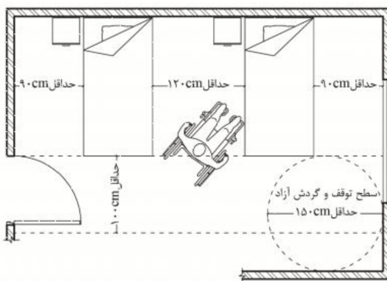
شکل شماره ۹۱: فضای آزاد در اتاق دو یا چند نفره بستری
