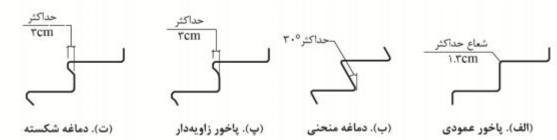
شکل شماره ۵۷: دماغه و پاخور پله‌ها
