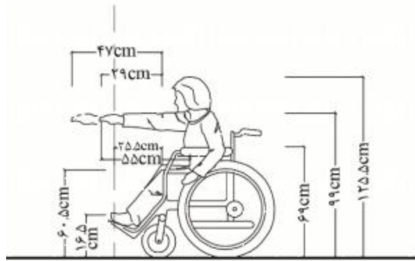
شکل شماره ۴: اندازه‌ها و دسترسی‌های زن معلول در حرکت به جلو
