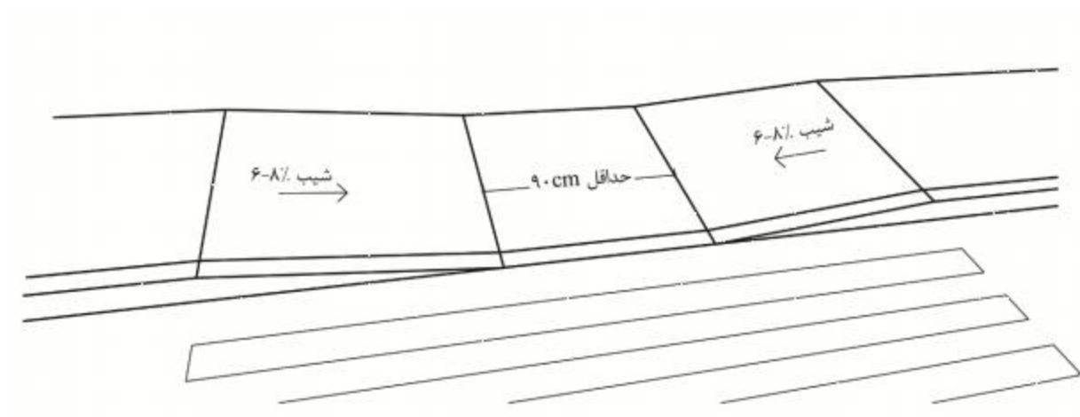
شکل شماره ۳۳: رمپ جدول موازی
