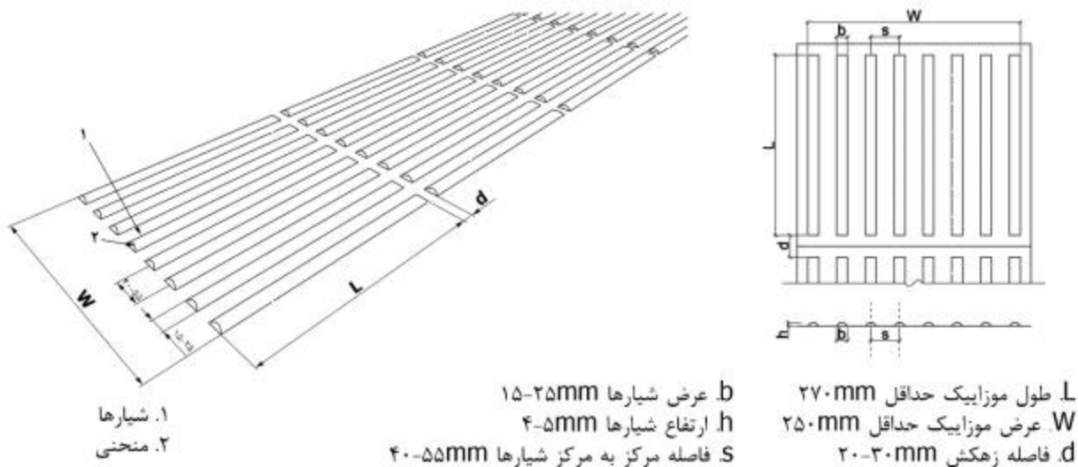
شکل شماره ۲۱: چیدمان، فواصل و ابعاد کفپوش شیاردار منحنی
