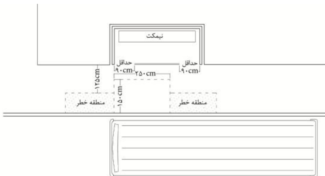
شکل شماره ۴۰: ایستگاه اتوبوس سربو شیده
