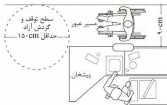
شکل شماره ۹۲: مسیر عبور و توقف جلوی پیشخان فروشگاه
