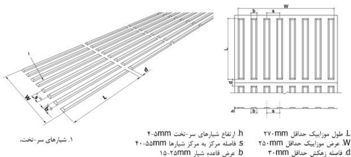
شکل شماره ۲۲: چیدمان، فواصل و ابعاد کفپوش شیاردار سر-تخت
