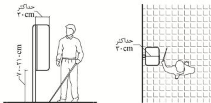
شکل شماره ۳۰: پیش‌آمدگی اشیای نصب شده روی پایه یا ستون
