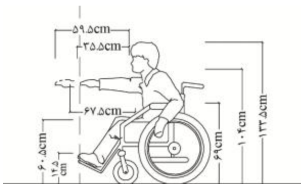
شکل شماره ۲: اندازه‌ها و دسترسی‌های افراد معلول در حرکت به جلو
