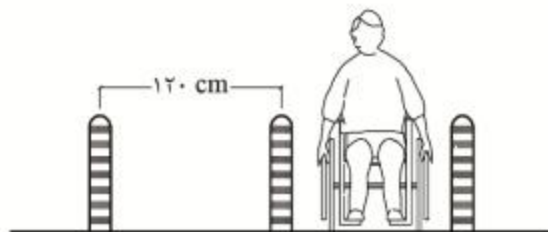
شکل شماره ۲۶: فاصله بین پست‌های ورودی
