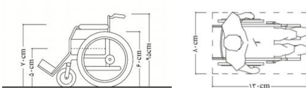
شکل شماره ۱: ابعاد استاندارد صندلی چرخدار
