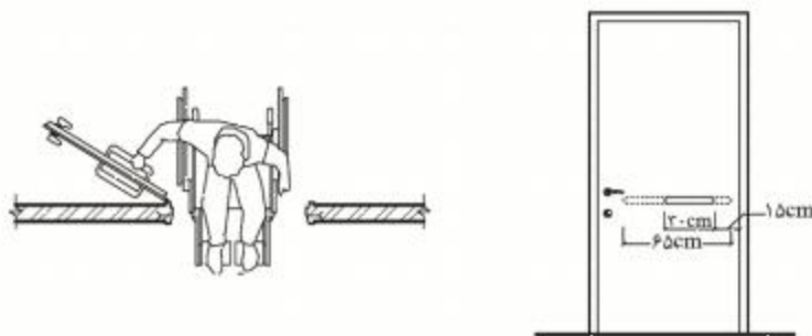
شکل شماره ۷۳: ابعاد میل به دستگرد کمکی روی درب
