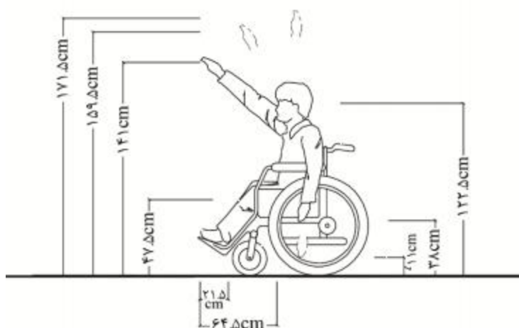
شکل شماره ۳: اندازه‌ها و دسترسی‌های افراد معلول در حرکت به بالا
